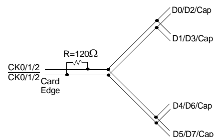
*Clock Net Wiring
