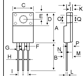
ITO-220
