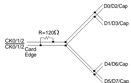
*Clock Net Wiring
