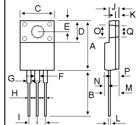
ITO-220
