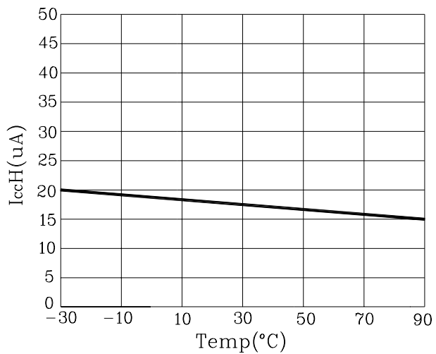
Fig. 3 I_{CC}H - Temp
