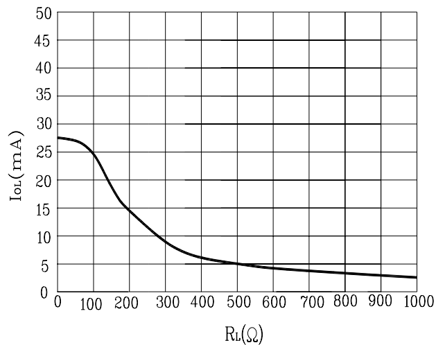
Fig. 4 I_{OL} - R_L
