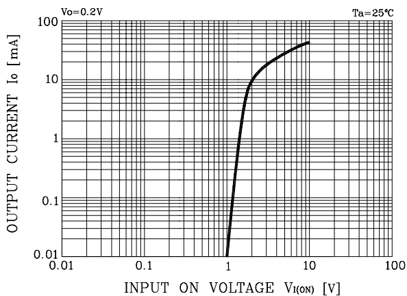
Fig. 3 G_1 - I_O
