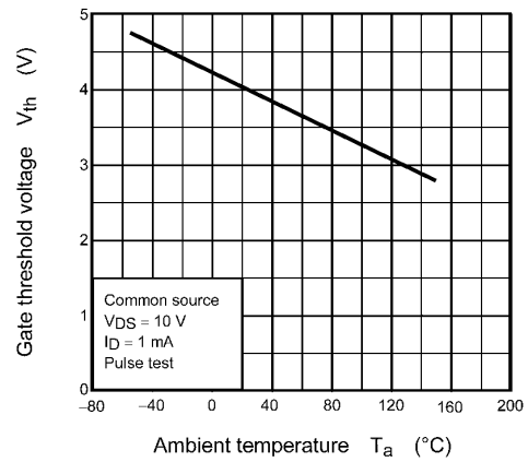
Fig. 8.10 V_{th} - T_a
