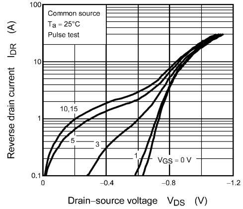
Fig. 8.8 I_{DR} - V_{DS}
