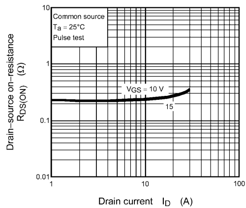
Fig. 8.6 R_{DS(ON)} - I_D
