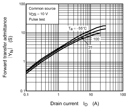
Fig. 8.5 |Y_{fs}| - I_D
