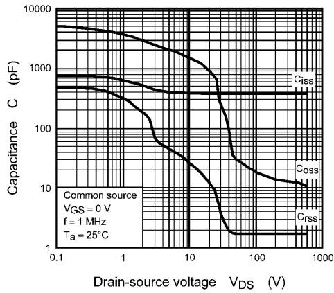
Fig. 8.9 C - V_{DS}
