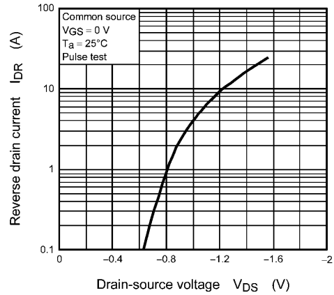
Fig. 8.8 I_{DR} - V_{DS}
