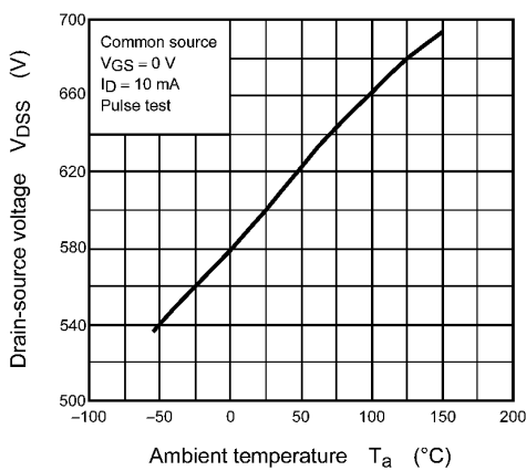
Fig. 8.5 V_{DS} - T_a
