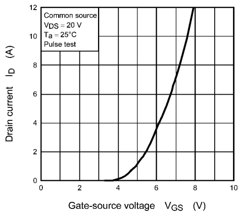
Fig. 8.3 I_D - V_{GS}
