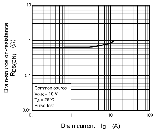
Fig. 8.6 R_{DS(ON)} - I_D
