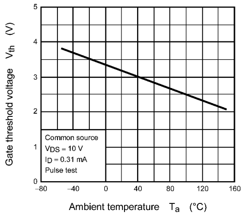
Fig. 8.11 V_{th} - T_a
