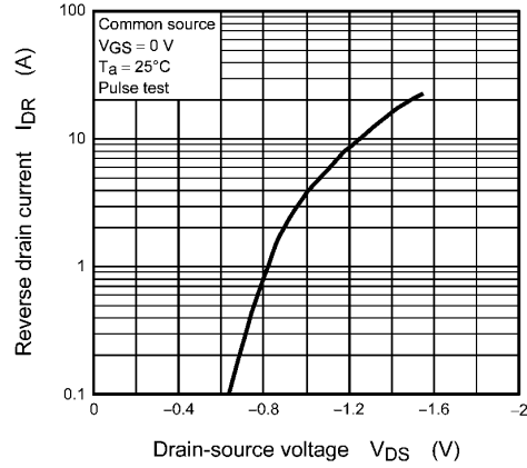
Fig. 8.8 I_{DR} - V_{DS}
