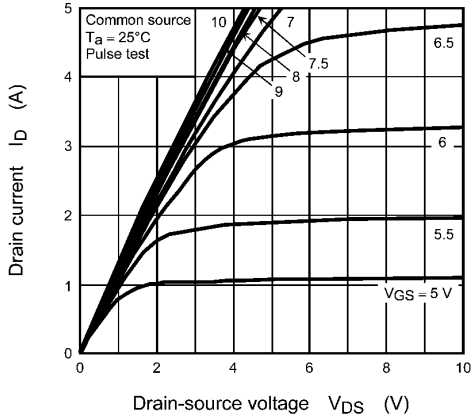
Fig. 8.1 I_D - V_{DS}
