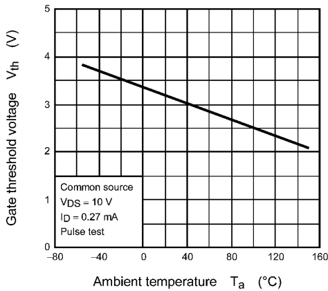
Fig. 8.11 V_{th} - T_a
