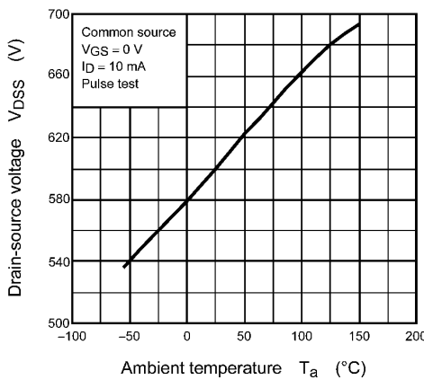
Fig. 8.5 V_{DSS} - T_a
