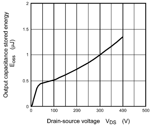
Fig. 8.10 E_{oss} - V_{DS}
