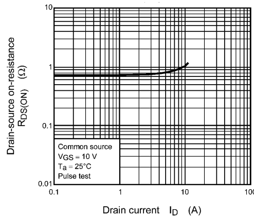
Fig. 8.6 R_{DS(ON)} - I_D
