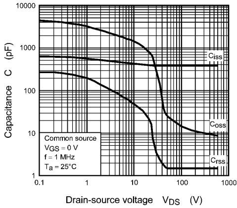
Fig. 8.9 C - V_{DS}
