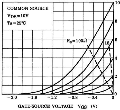
I_D - V_{GS}
