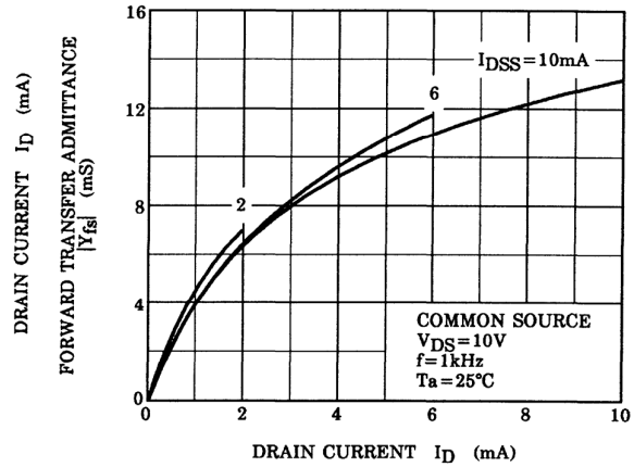
|Y_{fs}| - I_D
