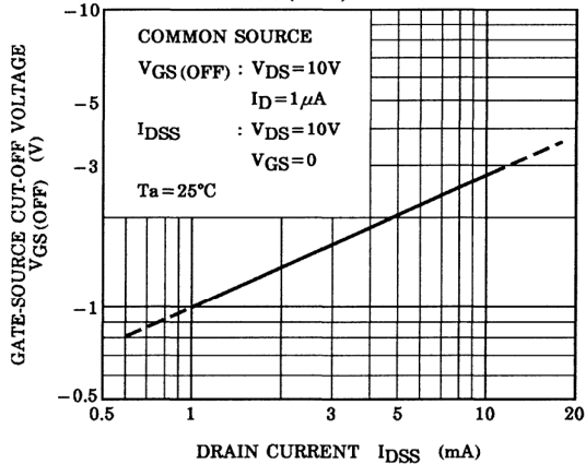
V_{GS(OFF)} - I_{DSS}
