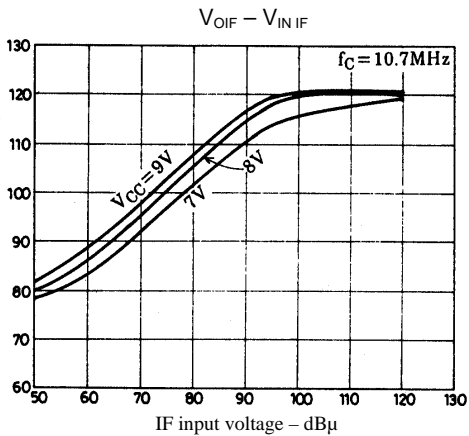
IF output - dBμ
