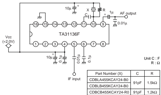
TA31136
