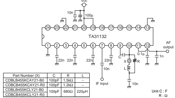
TA31132
