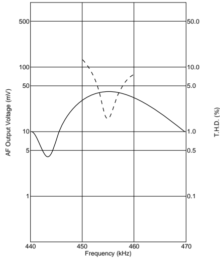
CDBC455KCAY40-R0
