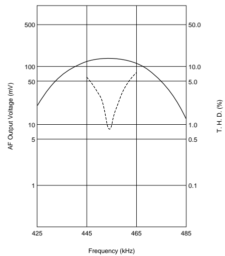
CDBC455KCLX39-R0
