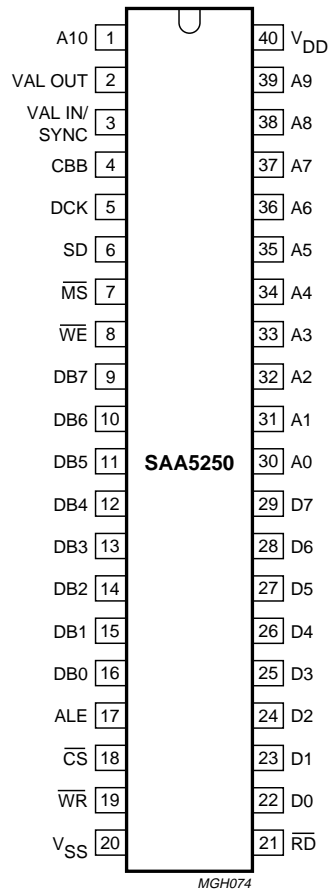
Fig.2 Pinning diagram.
