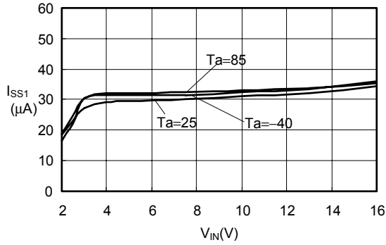
I_{SS1}-V_{IN} S-8520/21(Fosc:300 kHz)
