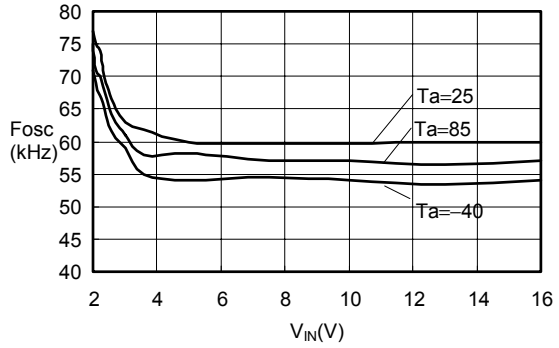
Fosc- V_{IN} S-8520/21(Fosc:60 kHz)
