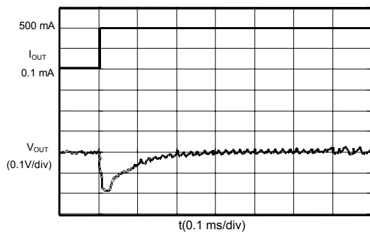
S-8520/1E33MC (VIN:4.0 V)
