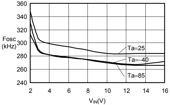
Fosc- V_{IN} S-8520/21(Fosc:300 kHz)
