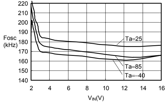
Fosc- V_{IN} S-8520/21(Fosc:180 kHz)
