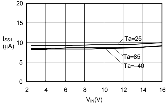
I_{SS1}-V_{IN} S-8520/21(Fosc:60 kHz)
