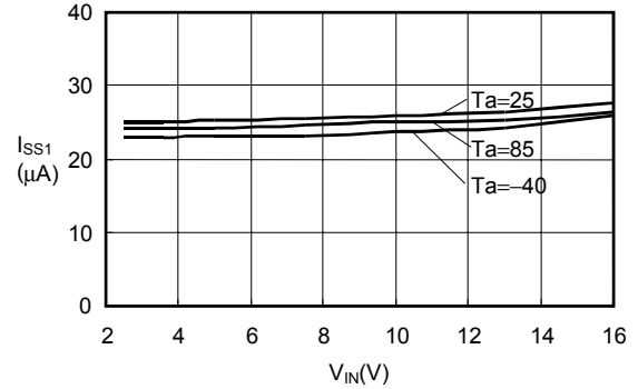
I_{SS1}-V_{IN} S-8520/21(Fosc:180 kHz)
