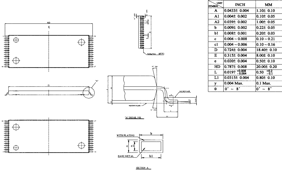
TSOP - 32
