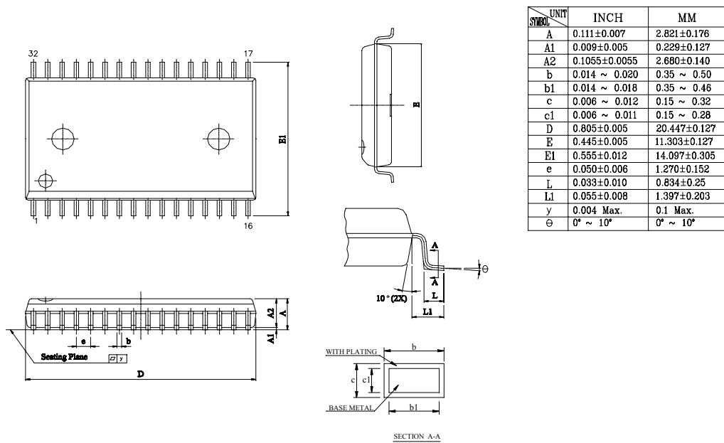
SOP - 32
