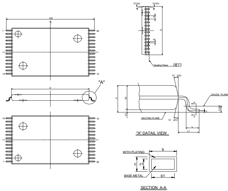
TSOP - 28
