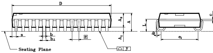
SOJ - 28
