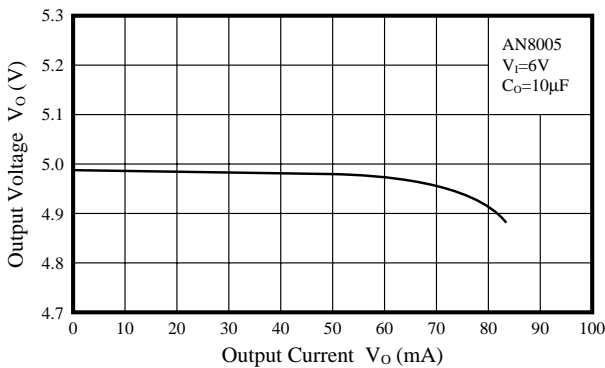
V_O - I_O
