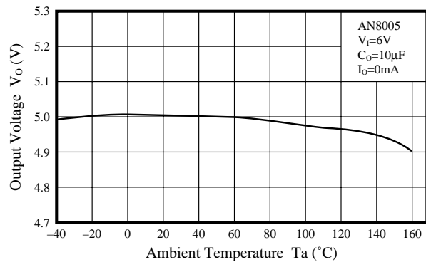
V_O - T_a
