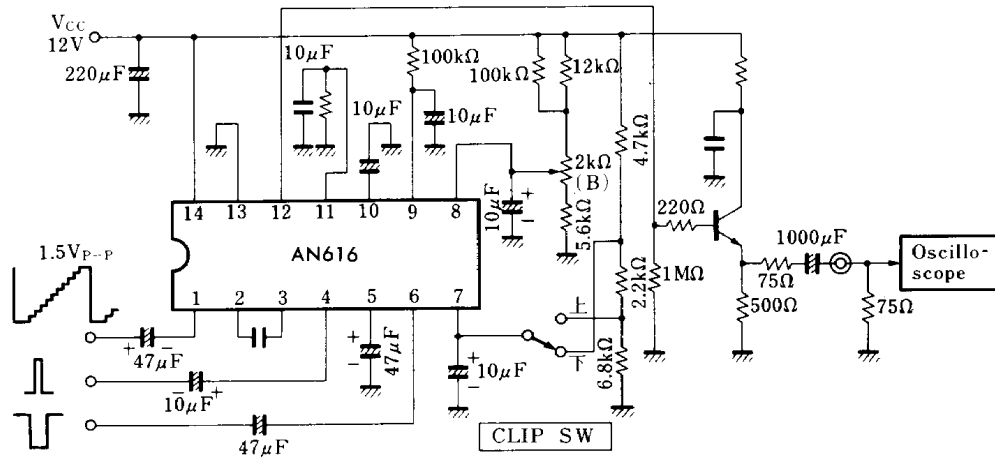
Test Circuit 3 ( V_{(3)} , V_{(4)} )
