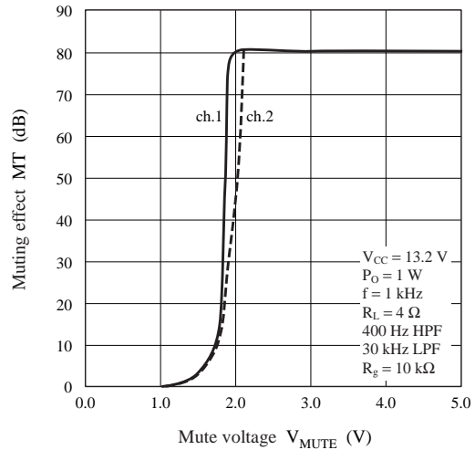
MT — V_{MUTE}
