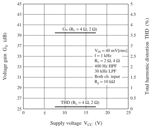
G_V , THD — V_{CC}
