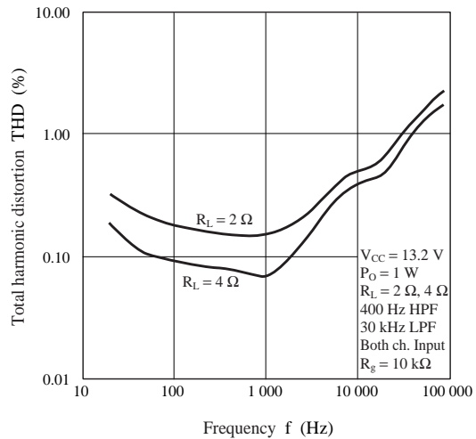
THD — f
