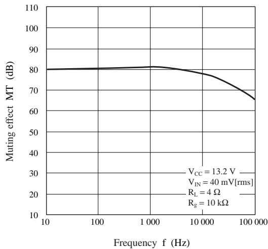
MT — f
