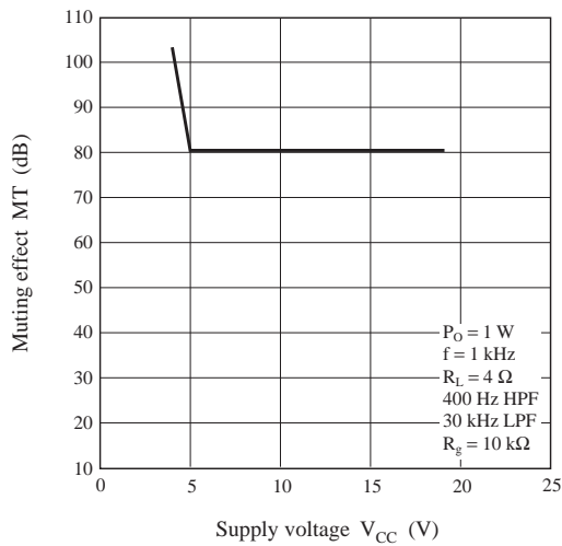
MT — V_{CC}
