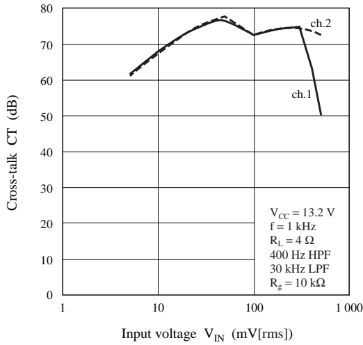
CT — V_{IN}
