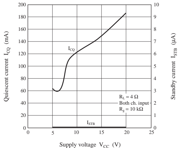
I_{CQ} , I_{STB} — V_{CC}
