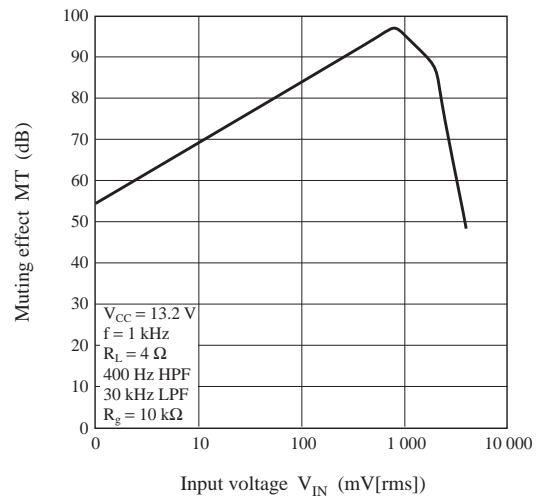
MT — V_{IN}
