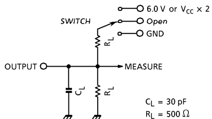
Fig.2 t_{pLH} , t_{pHL} , t_w , t_s , t_h
