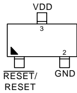
SOT-23-3
