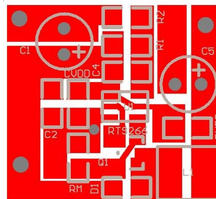
- Top Layer -
