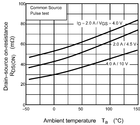
Fig. 7.6 R_{DS(ON)} - T_a
