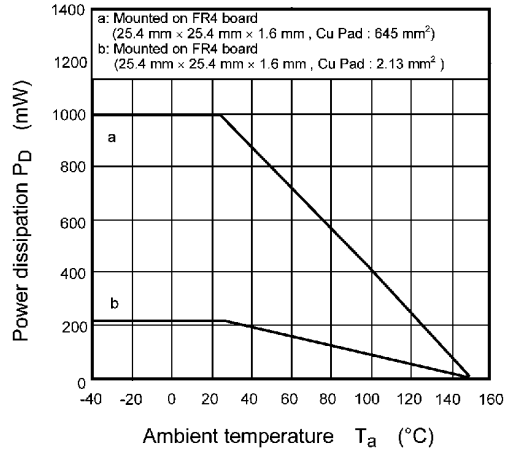
Fig. 7.14 P_D - T_a
