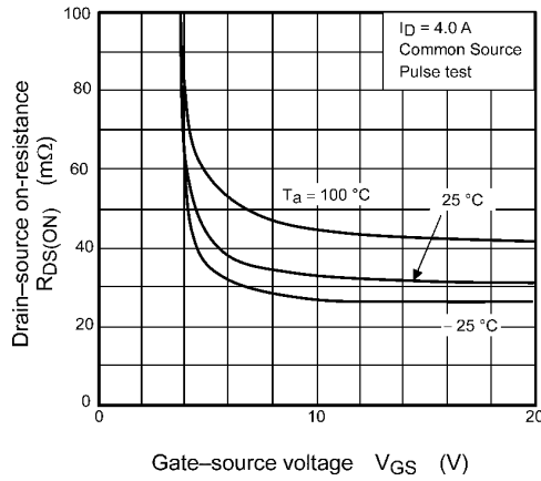
Fig. 7.4 R_{DS(ON)} - V_{GS}
