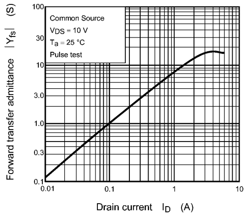
Fig. 7.8 |Y_{fs}| - I_D
