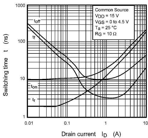
Fig. 7.11 t - I_D
