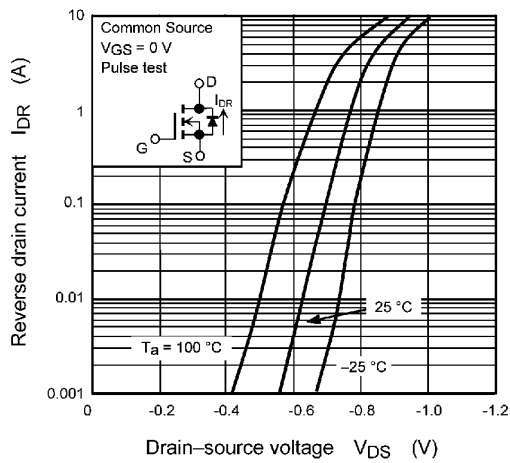
Fig. 7.9 I_{DR} - V_{DS}
