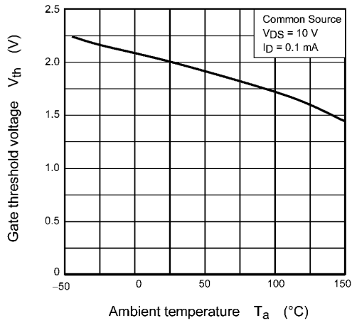
Fig. 7.7 V_{th} - T_a
