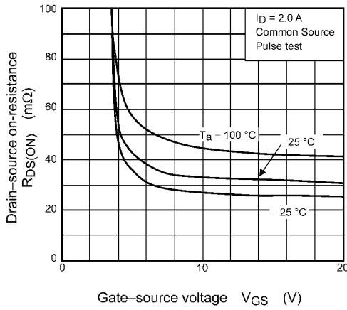
Fig. 7.3 R_{DS(ON)} - V_{GS}
