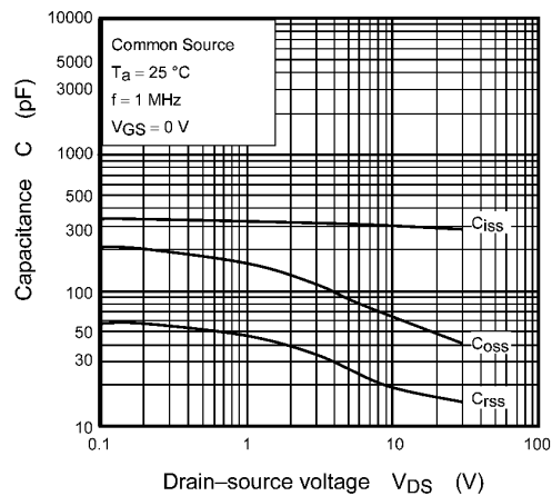
Fig. 7.10 C - V_{DS}
