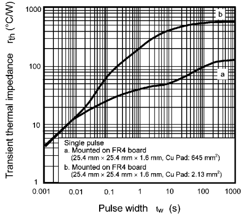
Fig. 7.13 r_{th} - t_w
