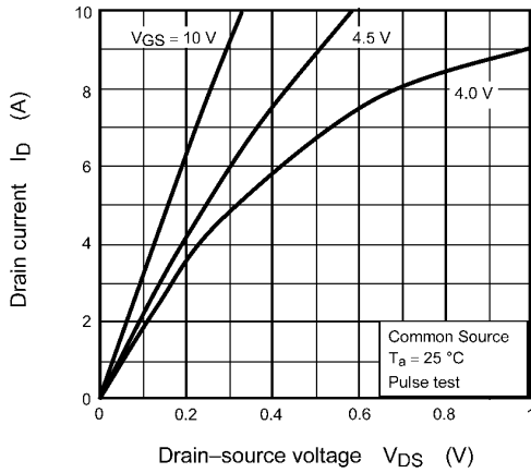
Fig. 7.1 I_D - V_{DS}
