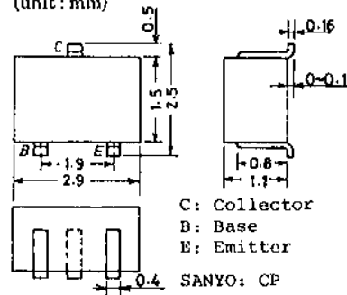
外形図 2018A (unit: mm)
