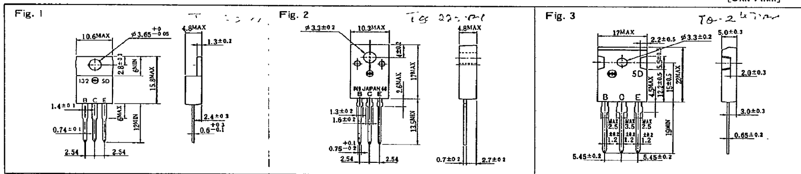
外形図 Outline Dimensions
