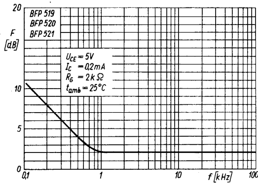
Zależność współczynnika szumów od częstotliwości F = f(f)
