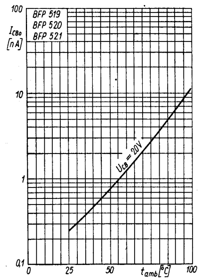
Zależność temperaturowa prądu zerowego I_{CBO} = f(t_{amb})
