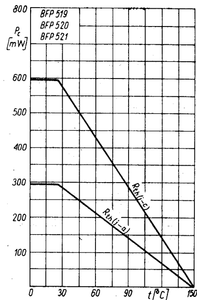
Zależność temperaturowa mocy strat P_c = f(t)
