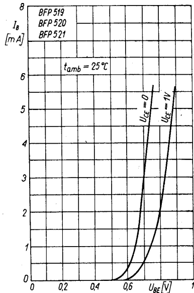
Charakterystyka wejściowa I_B = f(U_{BE}) ; U_{CE} — parametr
