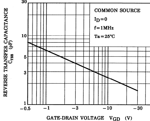
Crss - VGD
