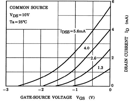
ID - VGS
