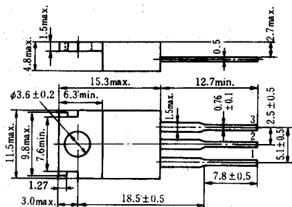
(JEDEC TO-220AB)
