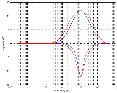
Figure 64 EQ Band 3 – EQ3BW=0, EQ3BW=1
