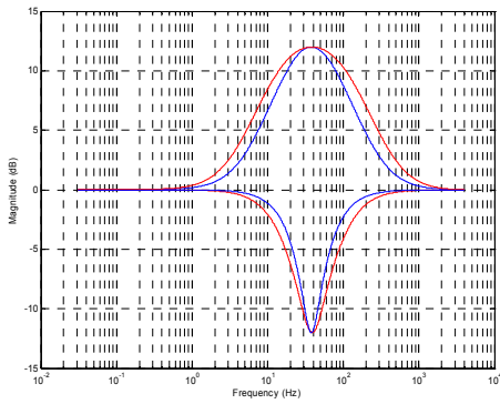
Figure 61 EQ Band 2 – EQ2BW=0, EQ2BW=1
