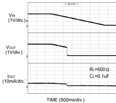
Fig.37 UVLO V_{IN} falling
