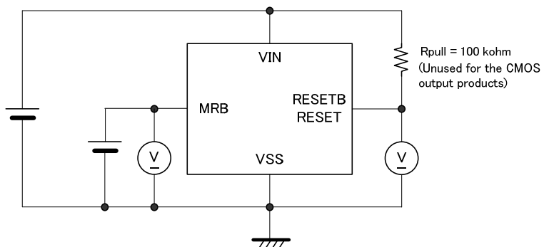
測定回路図⑥
