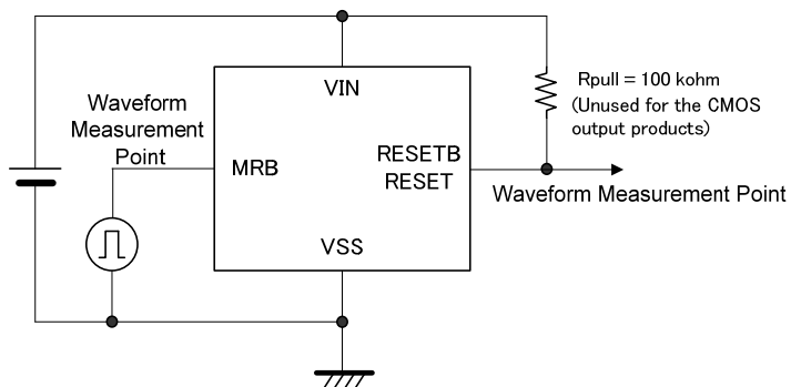
測定回路図⑦
