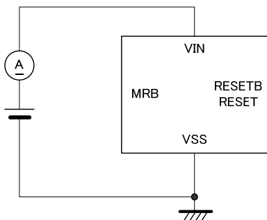
測定回路図②
