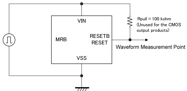
測定回路図④
