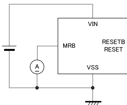
測定回路図⑥
