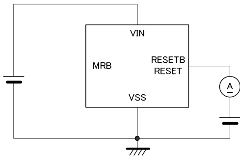
測定回路図③
