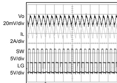
Fig.9 QLLM (Io=1.4A)
