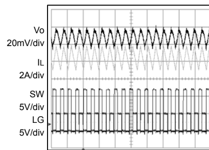
Fig.12 SLLM (Io=1.4A)
