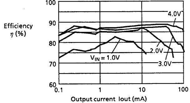
(d) Efficiency - Output current characteristics
