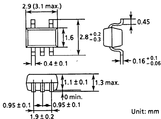
(1) SOT-23-5
