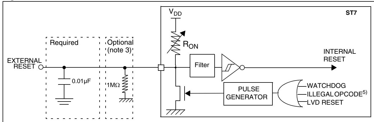
Figure 94. \overline{\text{RESET}} Pin Protection When LVD Is Enabled 1)2)3)4)
