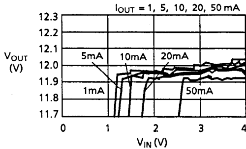
(b) V_{\text{IN}}-V_{\text{OUT}}
