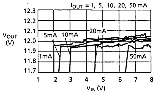
(b) V_{\text{IN}}-V_{\text{OUT}}
