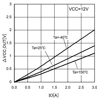
Fig.22 V(VCC-OUT)-Iout
