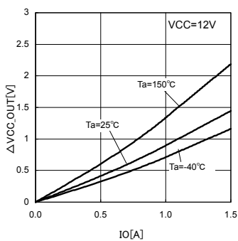
Fig.10 V(VCC-OUT)-Iout
