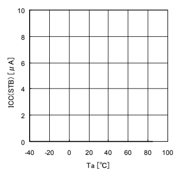
Fig.15 ICC(STB)-Ta
