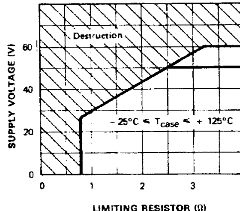
TDE1647,A - TDE1747
