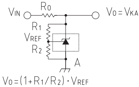
(2) V_{KA} \geq V_{REF} V_0 = V_{KA} = V_{REF}
