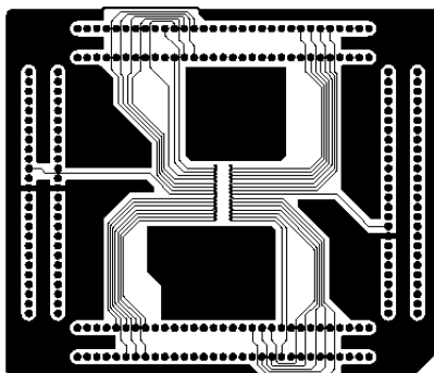
7 th layer
