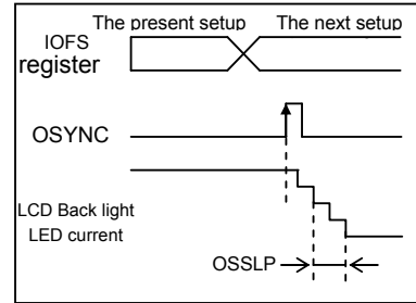
When OSYNCEN=0
