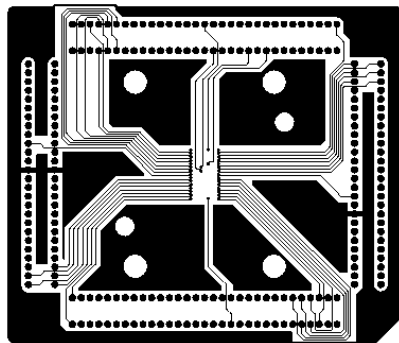
5 th layer
