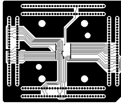
2 nd layer
