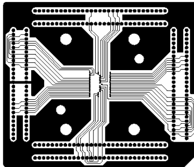
3 rd layer
