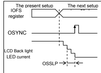
WHEN OSYNCEN=1
