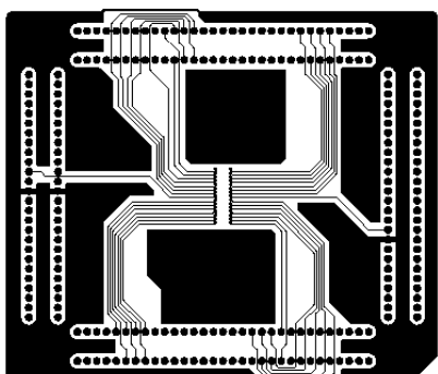
7 th layer
