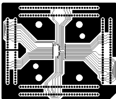
3 rd layer
