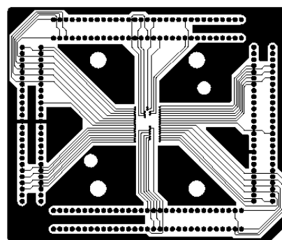
4 th layer
