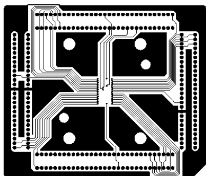
5 th layer
