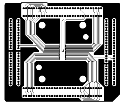
6 th layer
