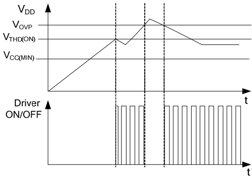
FIG.3 OVP case
