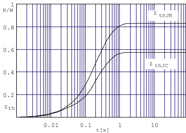
Transient thermal impedance per diode
