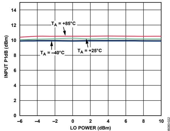
Figure 24. Input P1dB vs. LO Power
