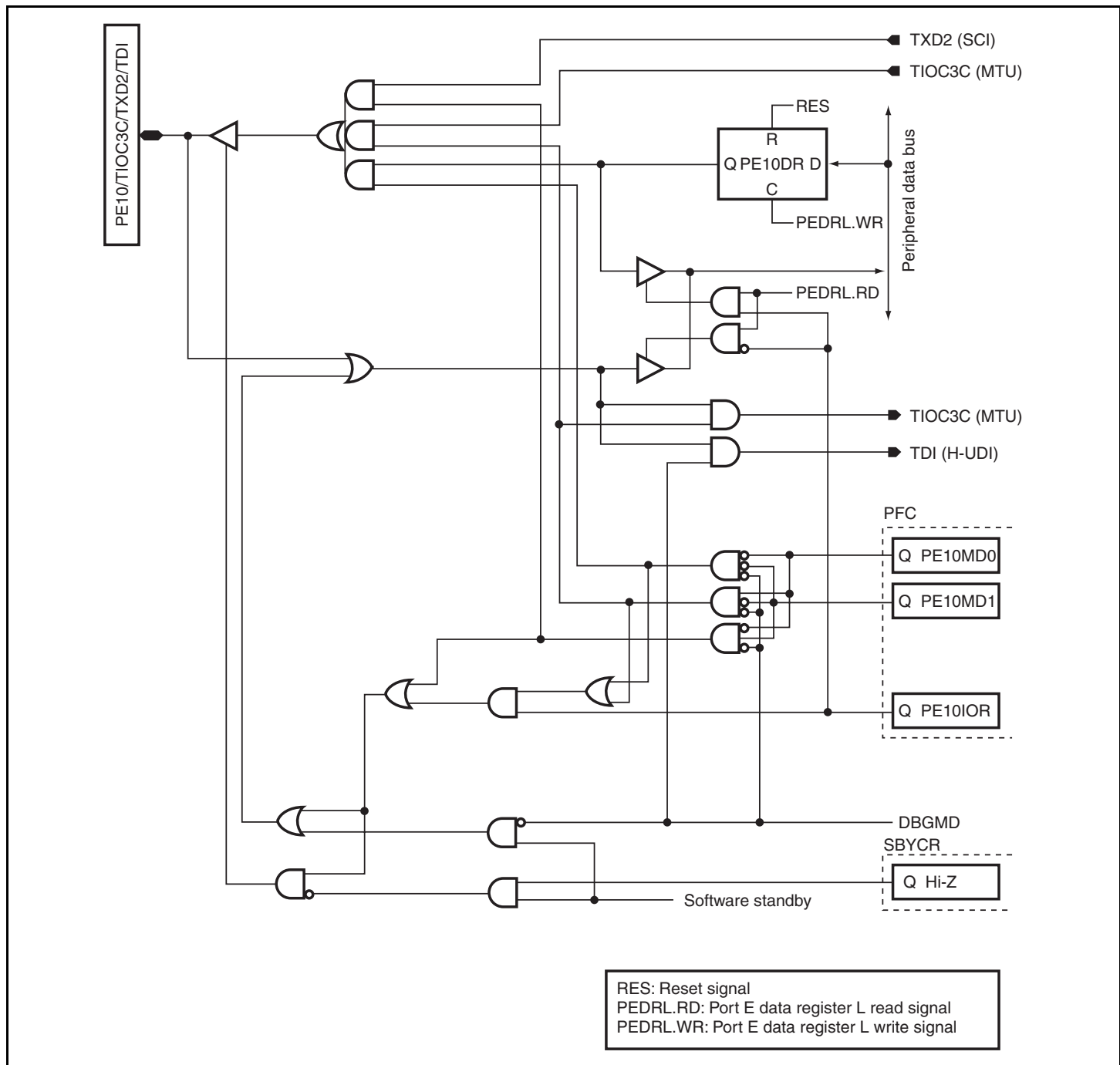
Figure D.54 PE10/TIOC3C/TXD2/TDI
