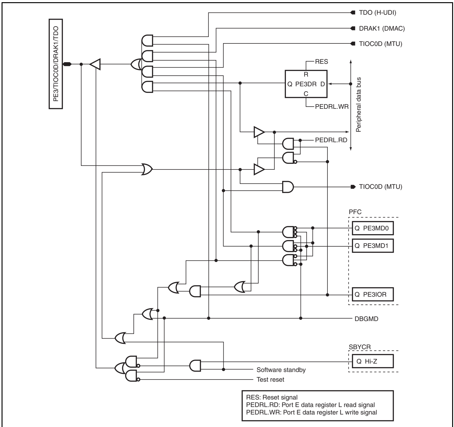
Figure D.45 PE3/TIOC0D/DRAK1/TDO
