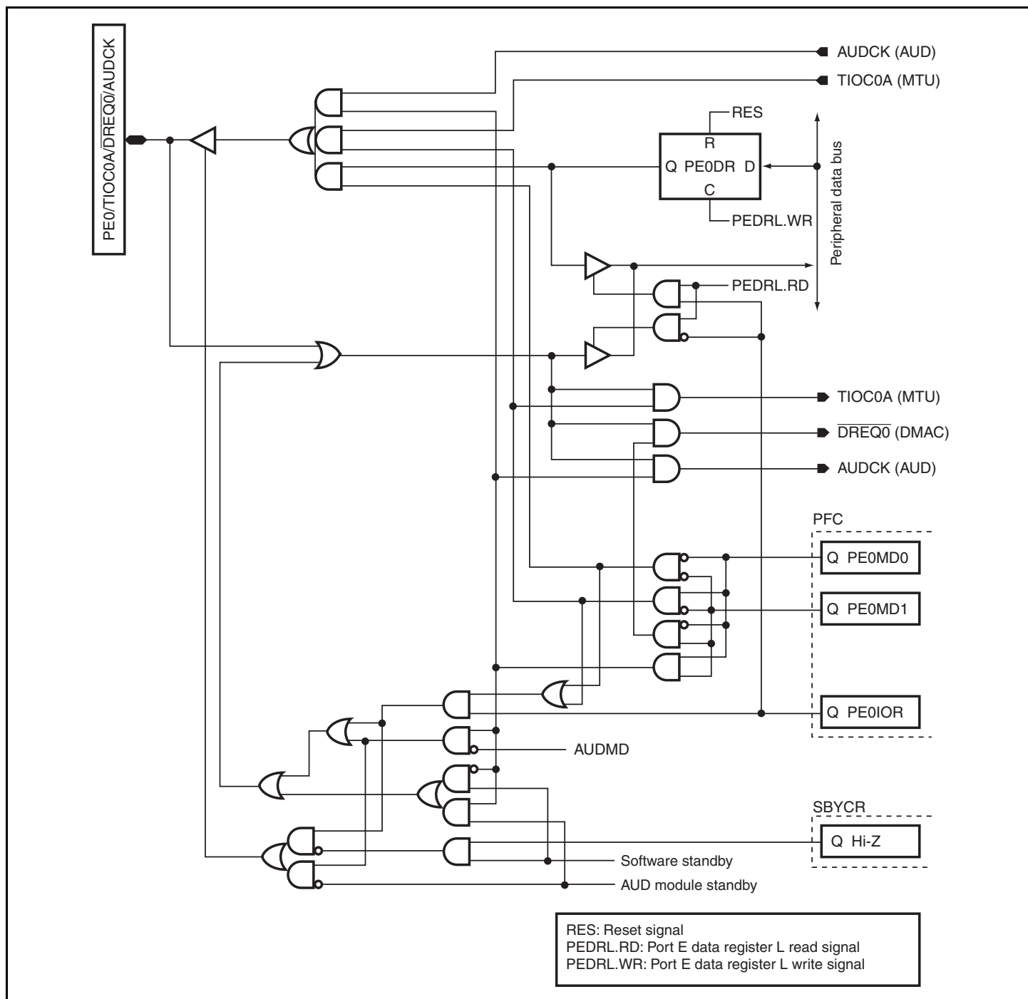
Figure D.46 PE0/TIOC0A/DREQ0/AUDCK
