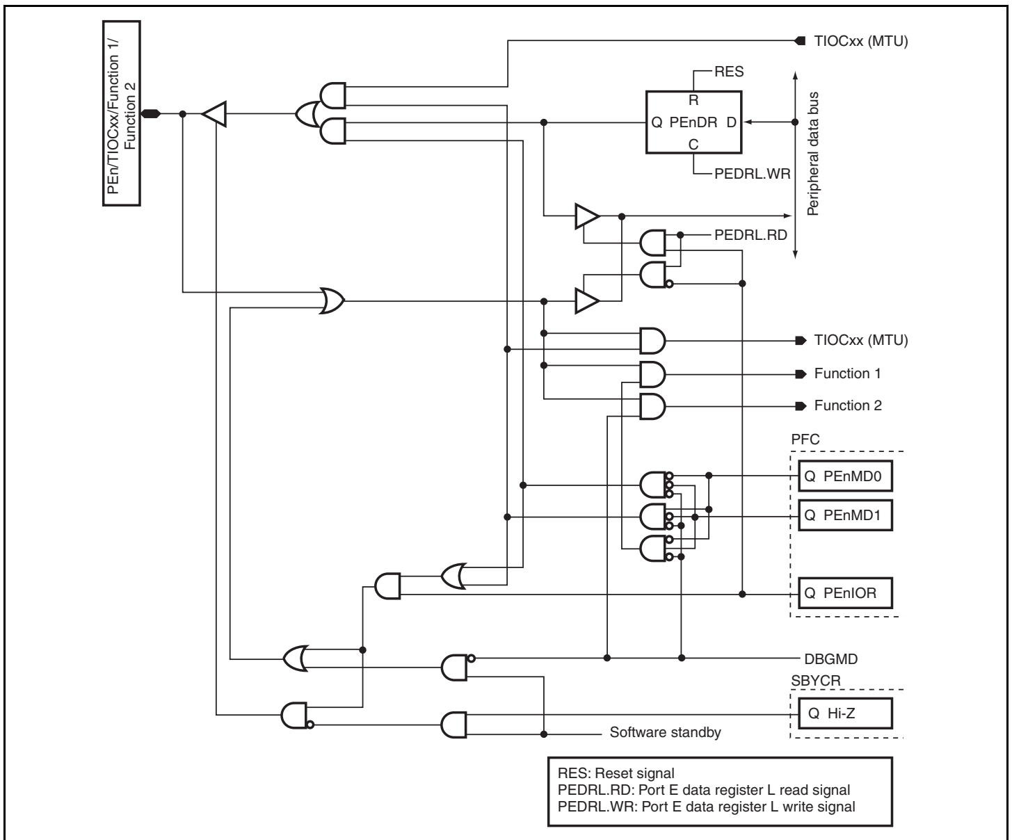
Figure D.43 PE n/TIOCxx/Function 1/Function 2
