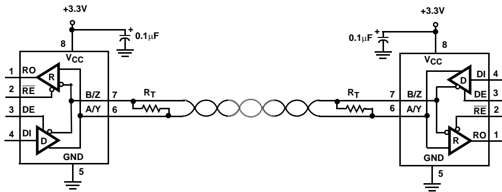
ISL83483, ISL83485
