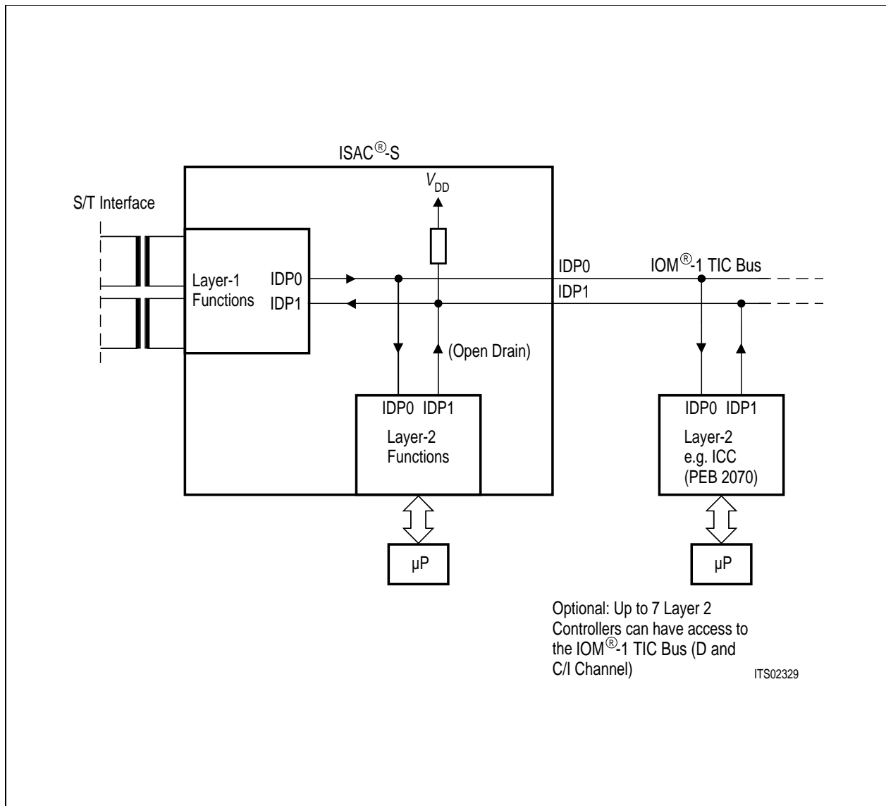
Figure 16 IOM ® -1 Data Ports 0, 1 (IOM ® -1)
