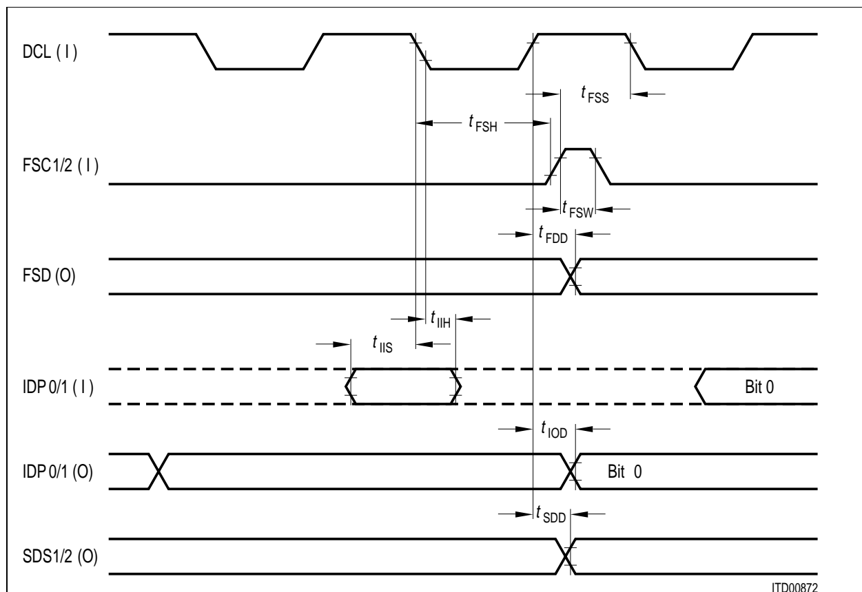
Figure 96 IOM ® Timing (LT-S, LT-T, NT mode)
