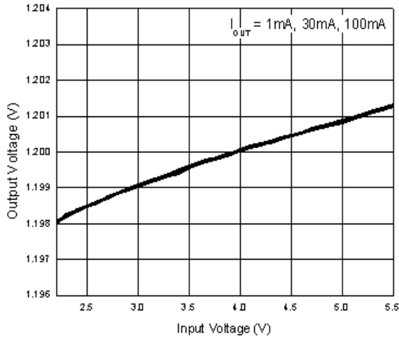
Fig. 7 Output Voltage VS Input Voltage (1.2V)
