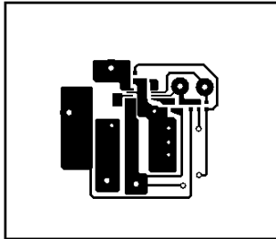
Fig. 35. Top layer
