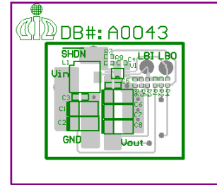
Fig. 37. Placement
