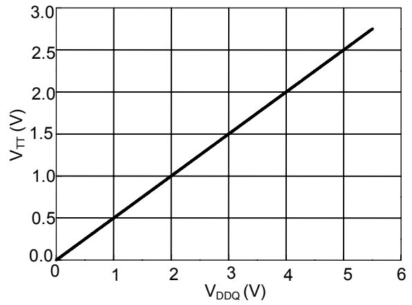
Fig. 6 V TT vs. V DDQ
