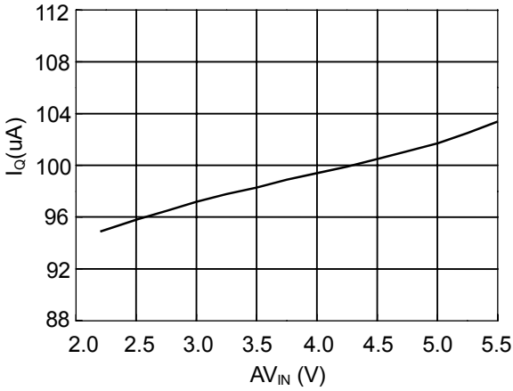
Fig. 1 I q vs. AV IN in Shutdown
