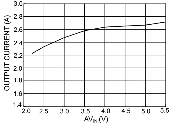
Fig.13 Maximum Sinking Current vs. AV IN (V DDQ =1.8V)
