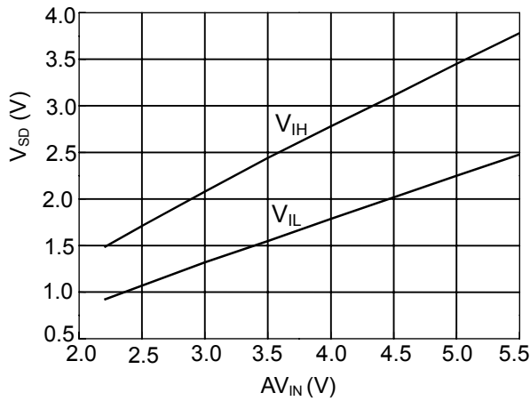
Fig. 3 AV IN vs. V SD
