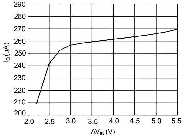
Fig. 2 I q vs. AV IN
