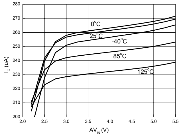
Fig.15 I Q vs. AV IN
