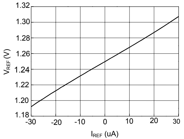
Fig. 4 V REF vs. I REF
