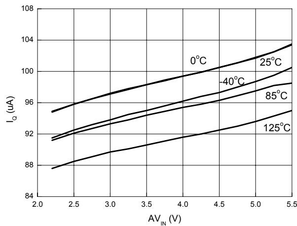
Fig.14 I Q vs. AV IN in Shutdown
